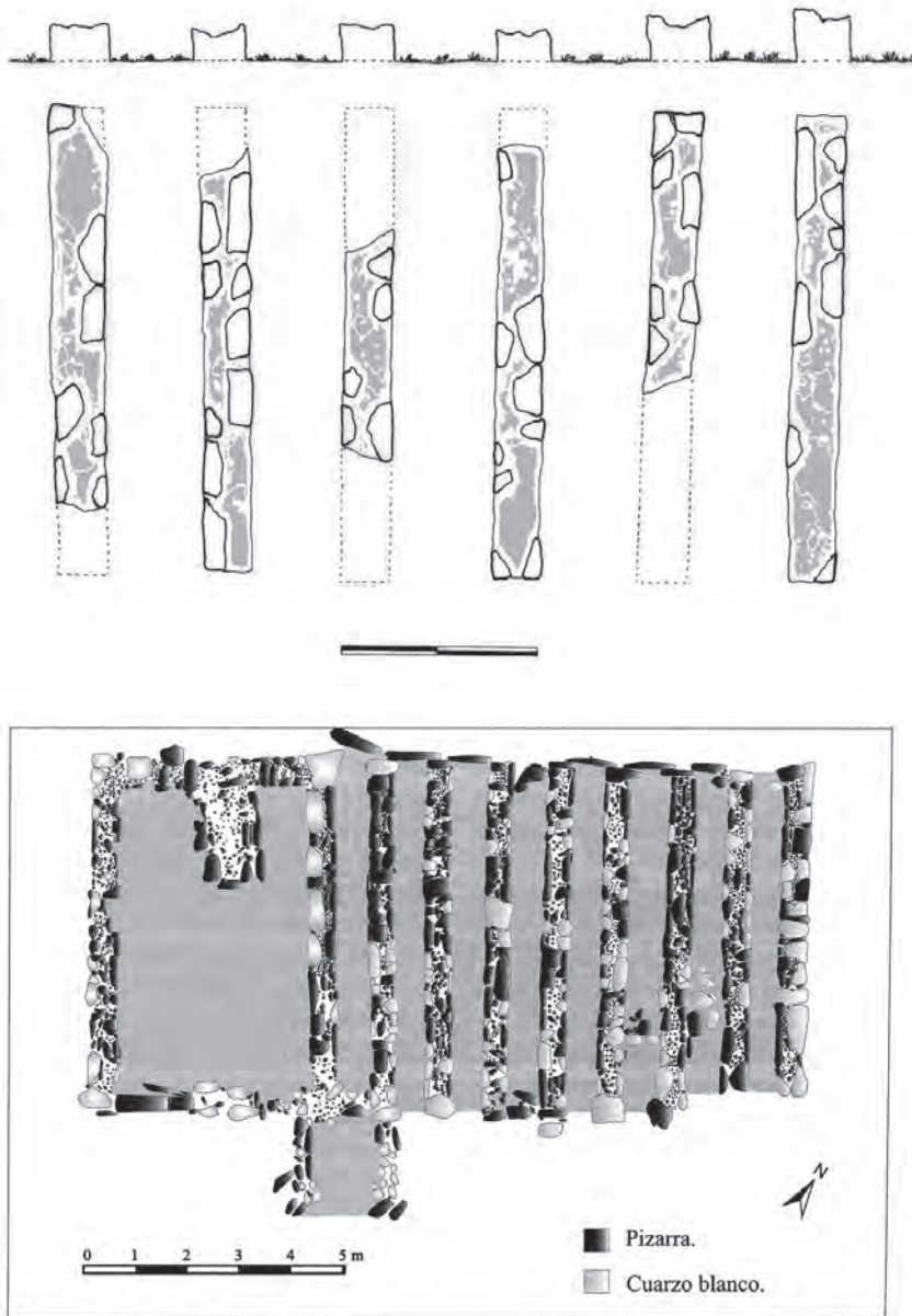
Fig. 3. Planta del horreum de la villa hispanorromana de Los Términos (Monroy, Cáceres). Imagen: P. J. Salido Domínguez.
